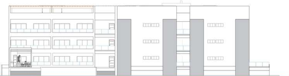
PLANO ELEVACIÓN LATERAL DERECHO
