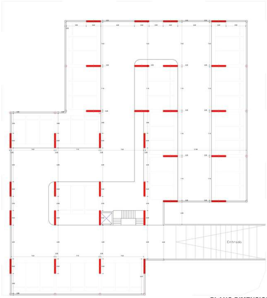
PLANO DIMENSIONADA CONJUNTO SOTANO
