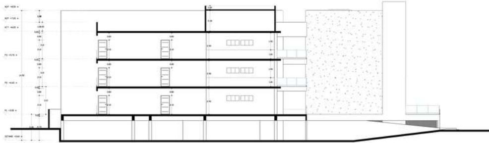
SECCIÓN A-A
