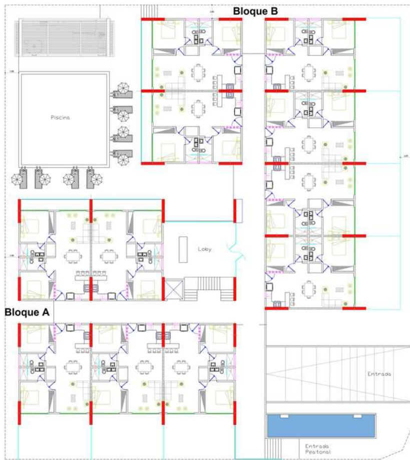
PLANO ARQUITECTONICO DE CONJUNTO 1ER NIVEL
